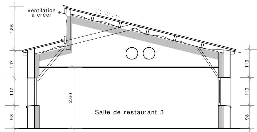
COUPE 3
