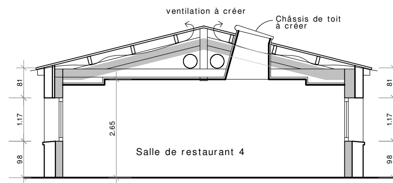
COUPE 4
