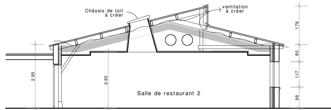
COUPE 2
