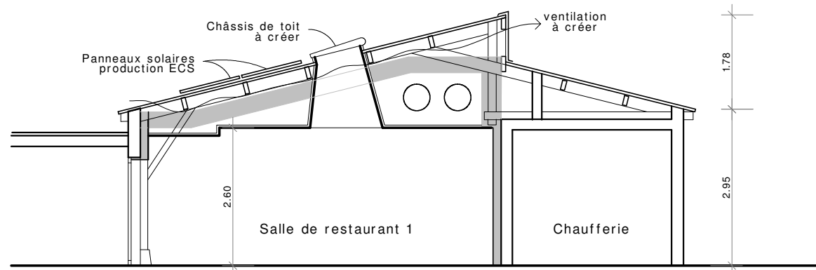
COUPE 1
